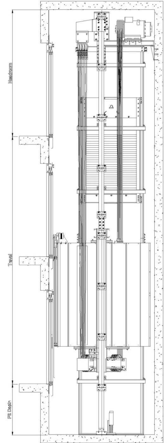
GIGAS 2500 Kg
