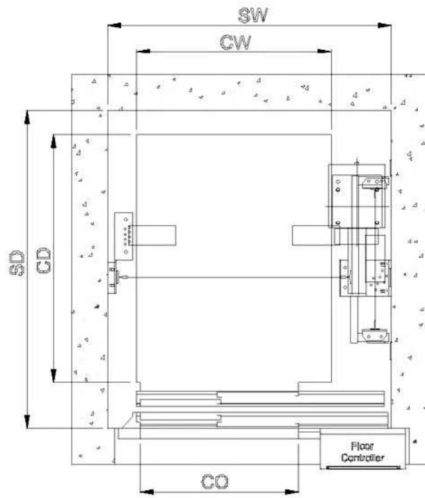
630 kg / 1 Side Opening Door
